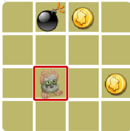
Figura 2: Vestimenta ELJuegoDeSbog.xml
